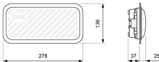
Montaje estanco
